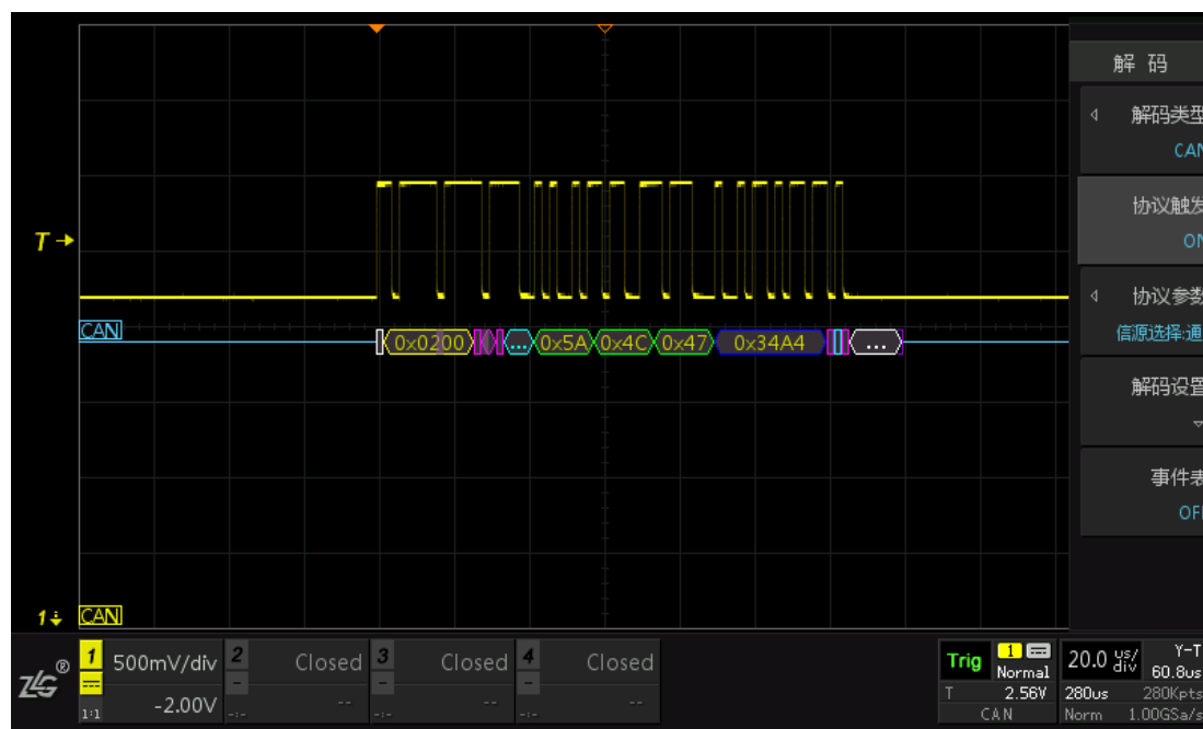
图 15.3 解码菜单
