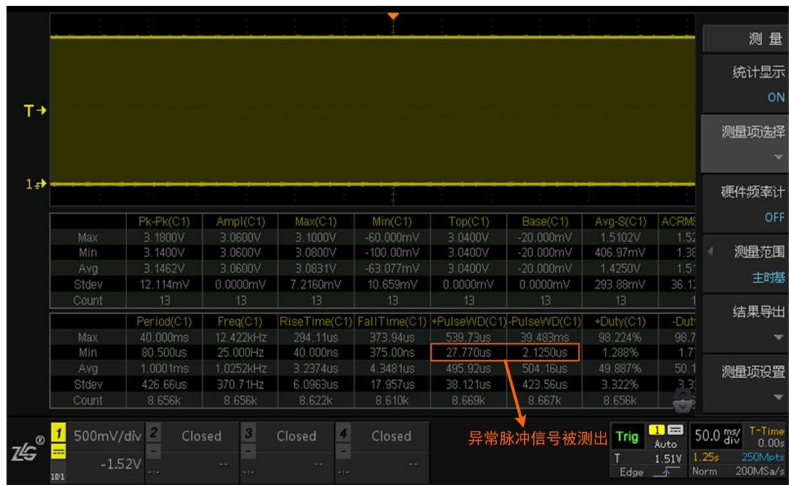
图 12.9 电压+时间综合测量
