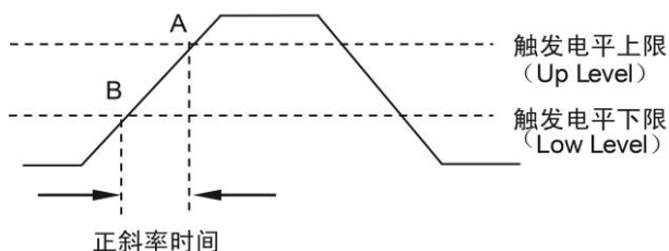
图 10.26 正斜率时间说明
