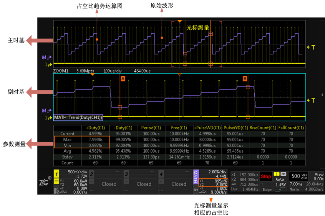
图 18.12 趋势运算界面
