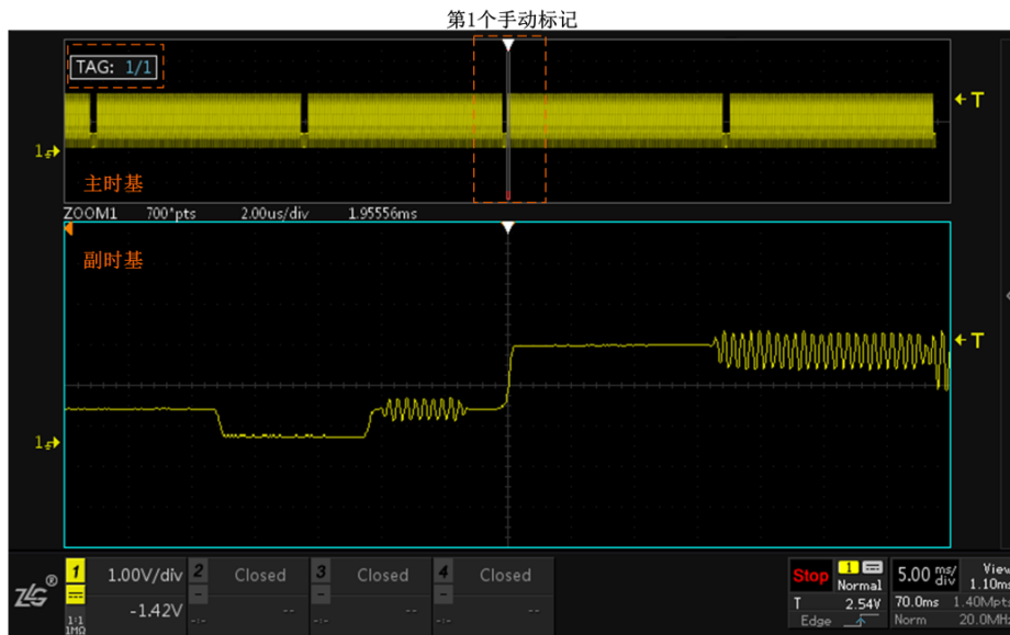
图 14.1 手动标注
