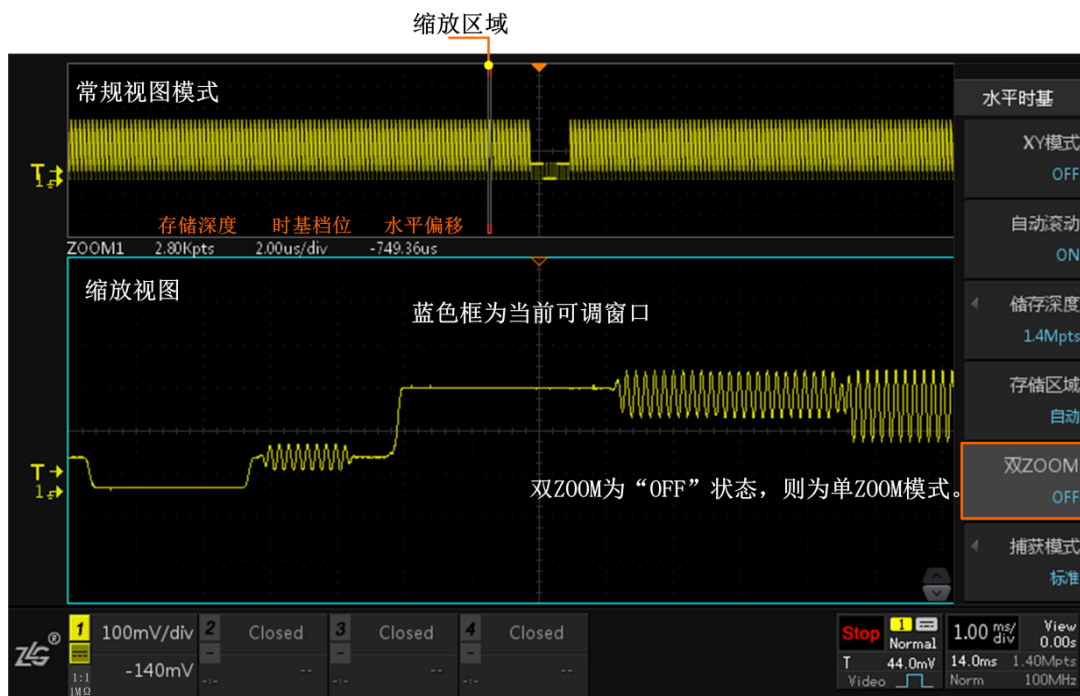
图 6.5 单 ZOOM 模式
