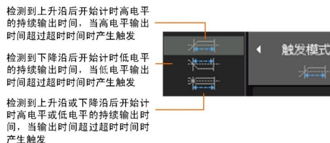
图 10.41 设置触发模式
