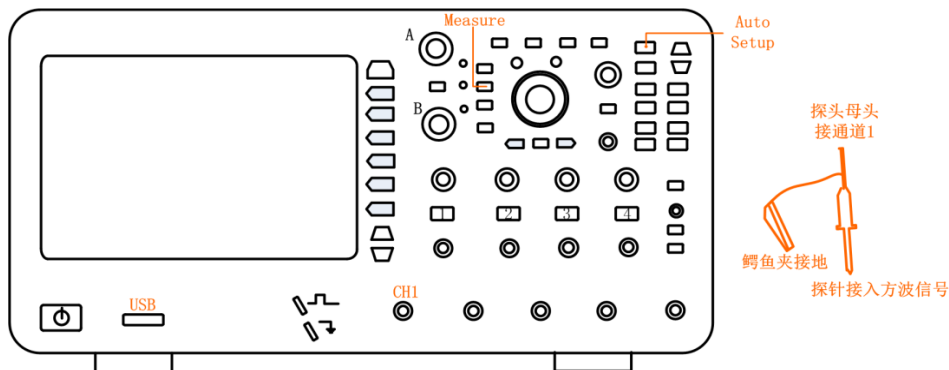
图 12.7 接入方波信号
