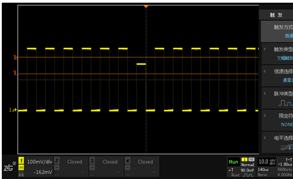
图 10.10 欠幅触发
