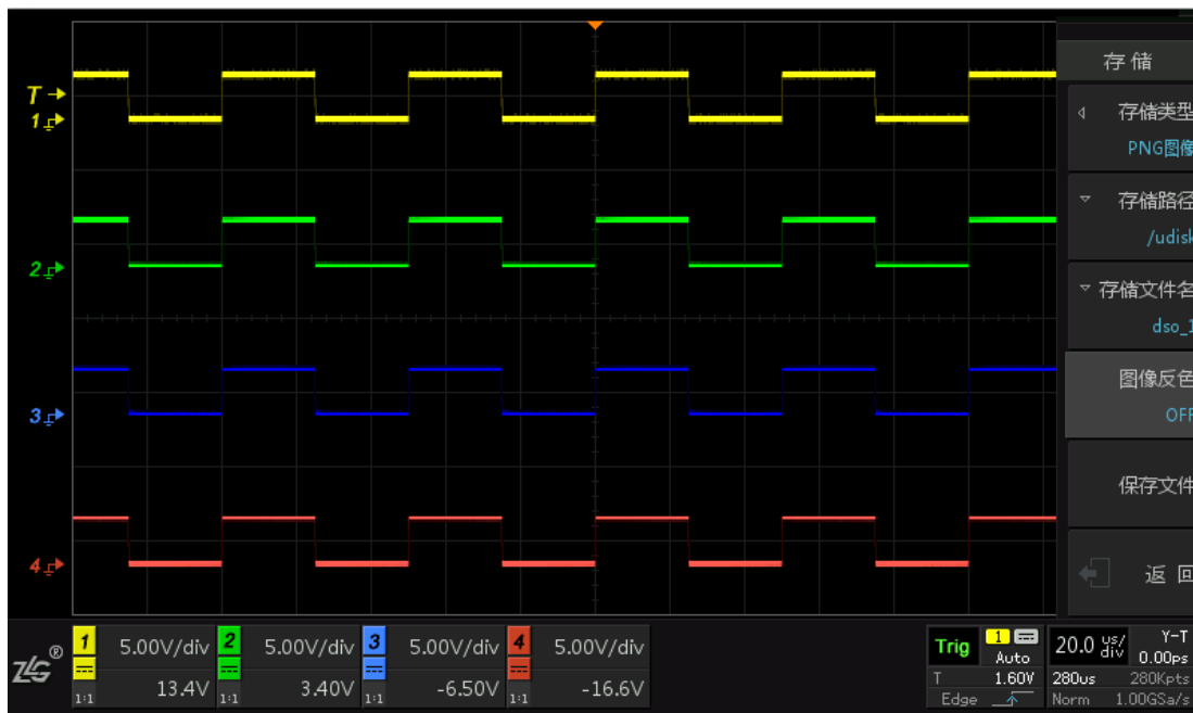
图 22.13 图像反相为“OFF”
