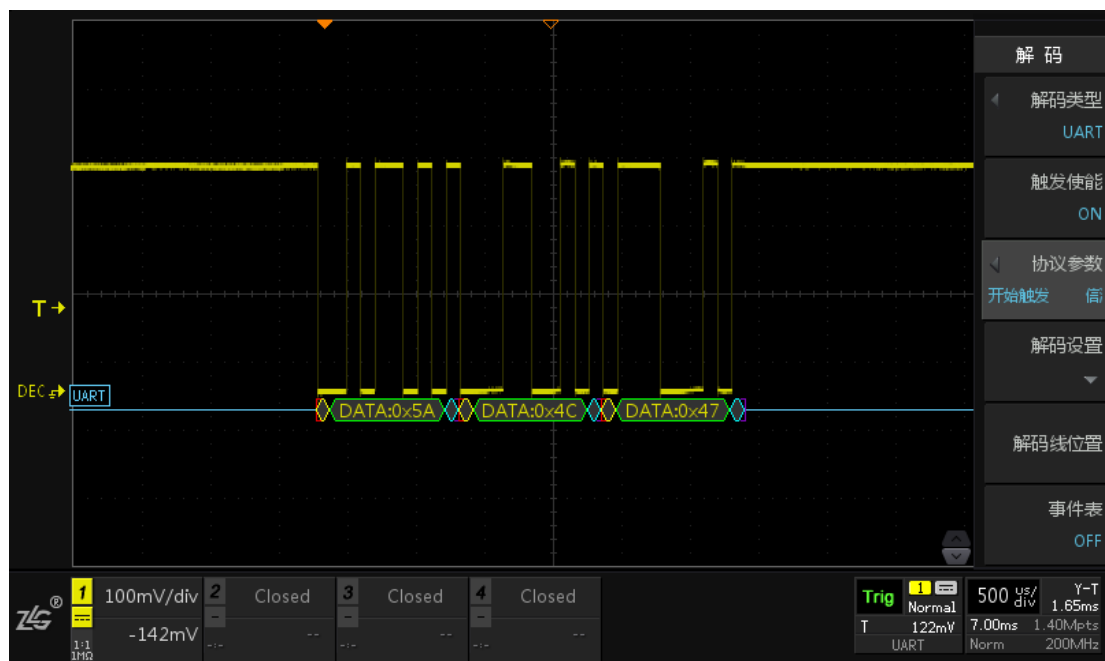
图 15.36 ZDS3000/4000 系列示波器的 UART 信号
