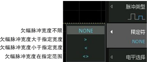
图 10.32 欠幅脉冲宽度限定
