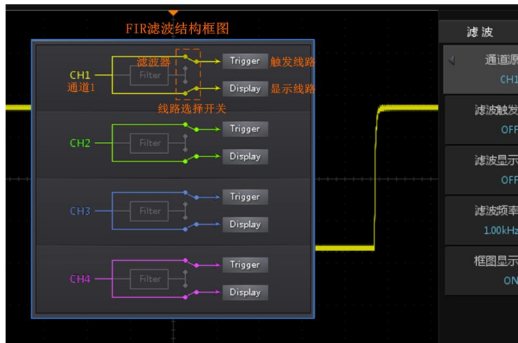
图 17.1 FIR 滤波界面
