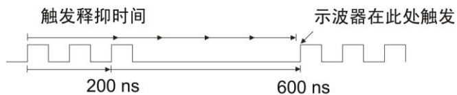
图 10.15 触发释抑时间设置
