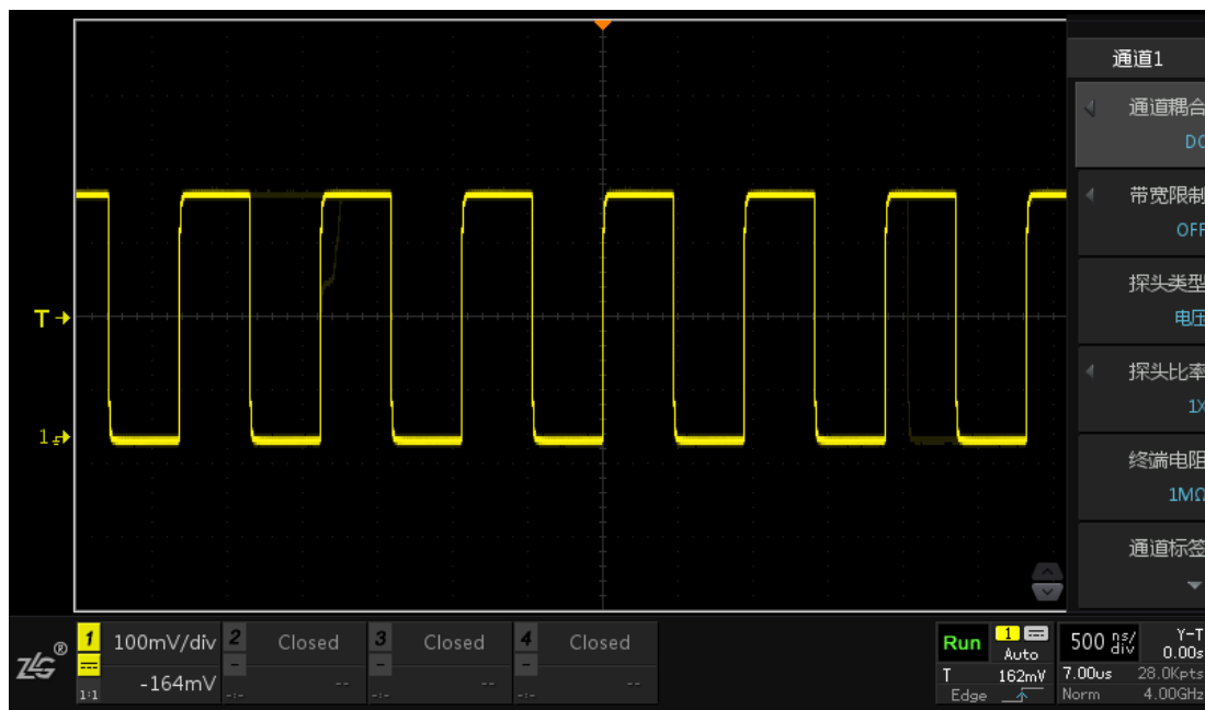
图 9.1 选中通道 1
