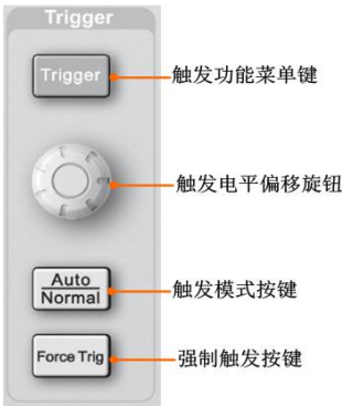
图 5.18 触发功能区
