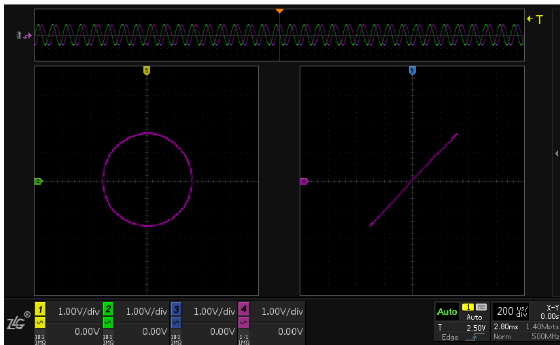
图 9.9 4 通道示波器 X-Y 模式
