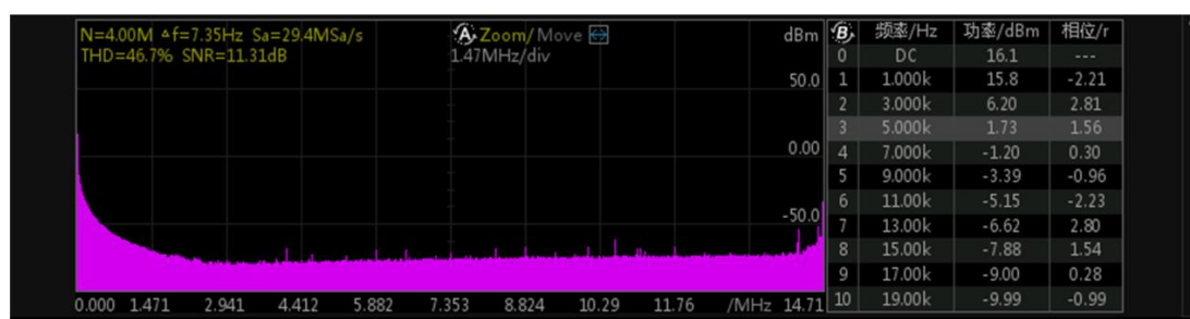
图 19.3 FFT 运算界面
