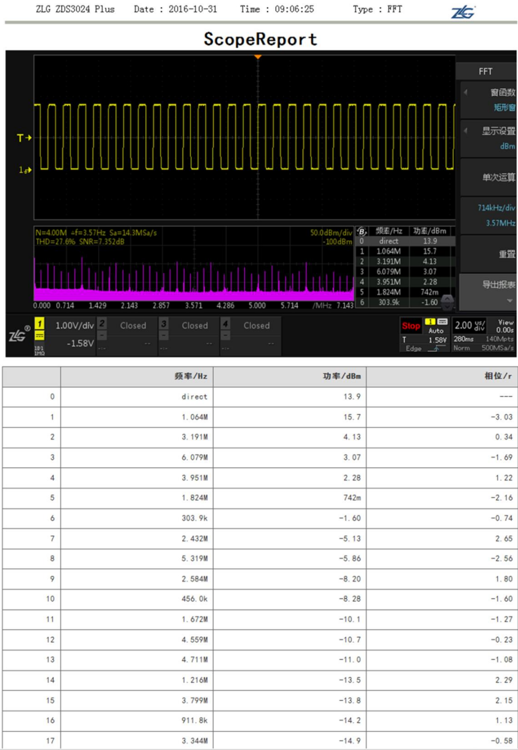
图 22.20 FFT 报表
