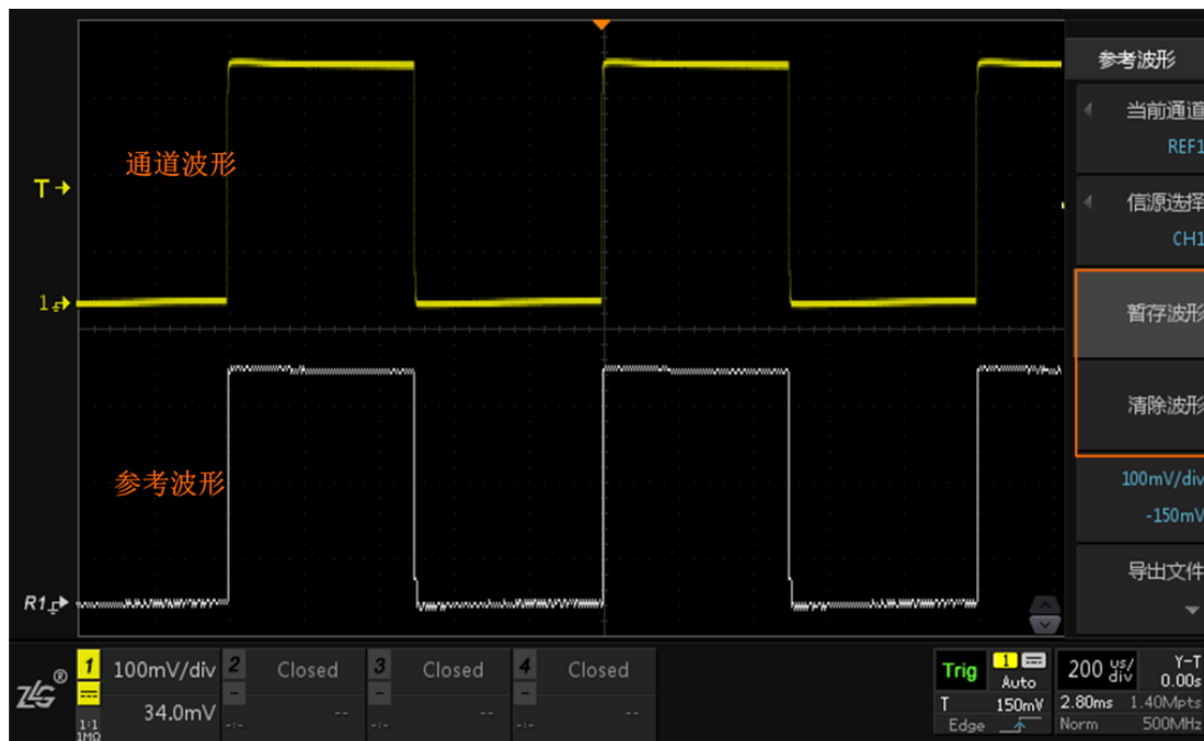
图 21.5 参考波形显示与对比
