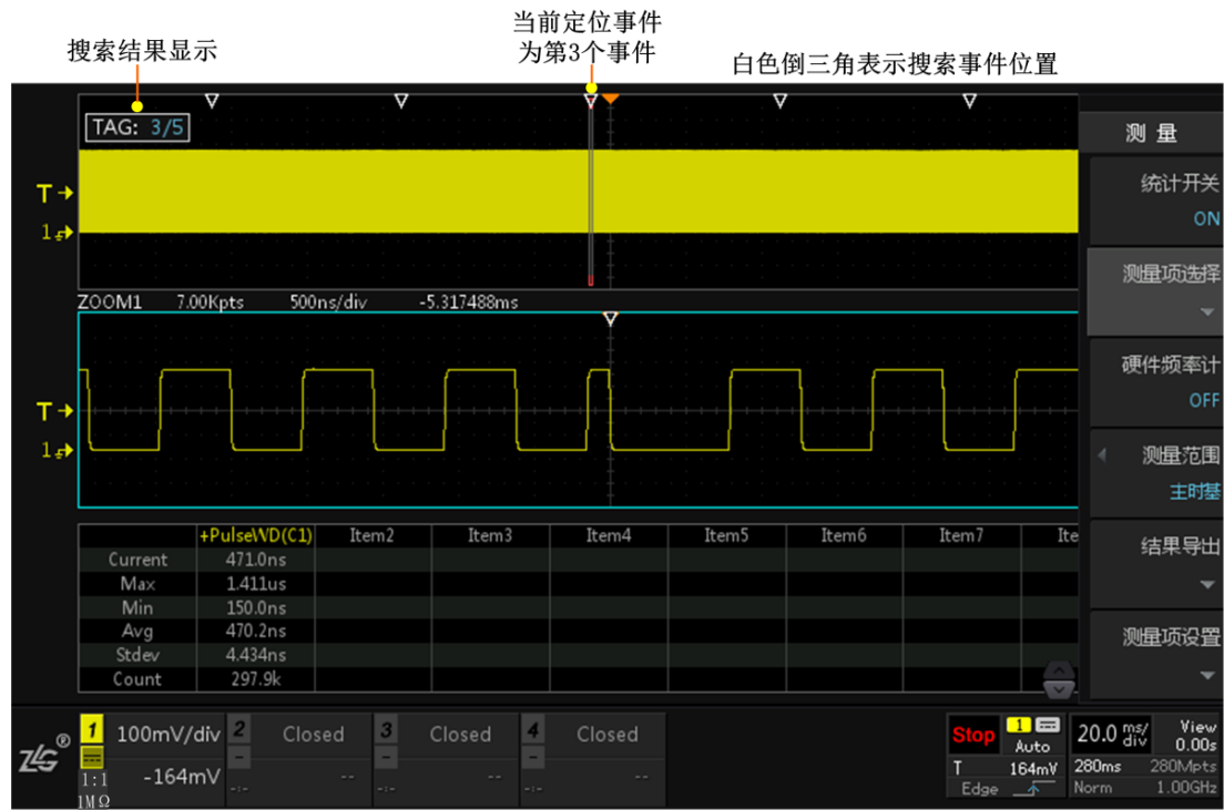
图 13.4 事件索引
