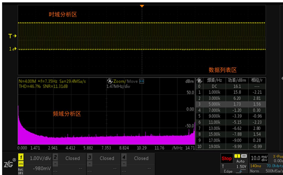
图 19.2 FFT 界面视图
