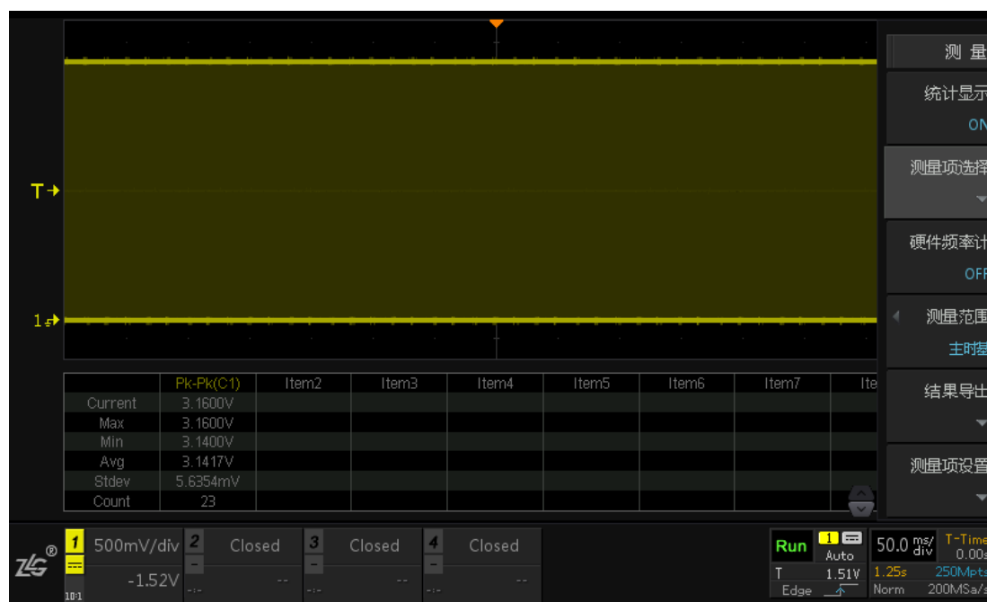
图 12.11 峰值测量结果
