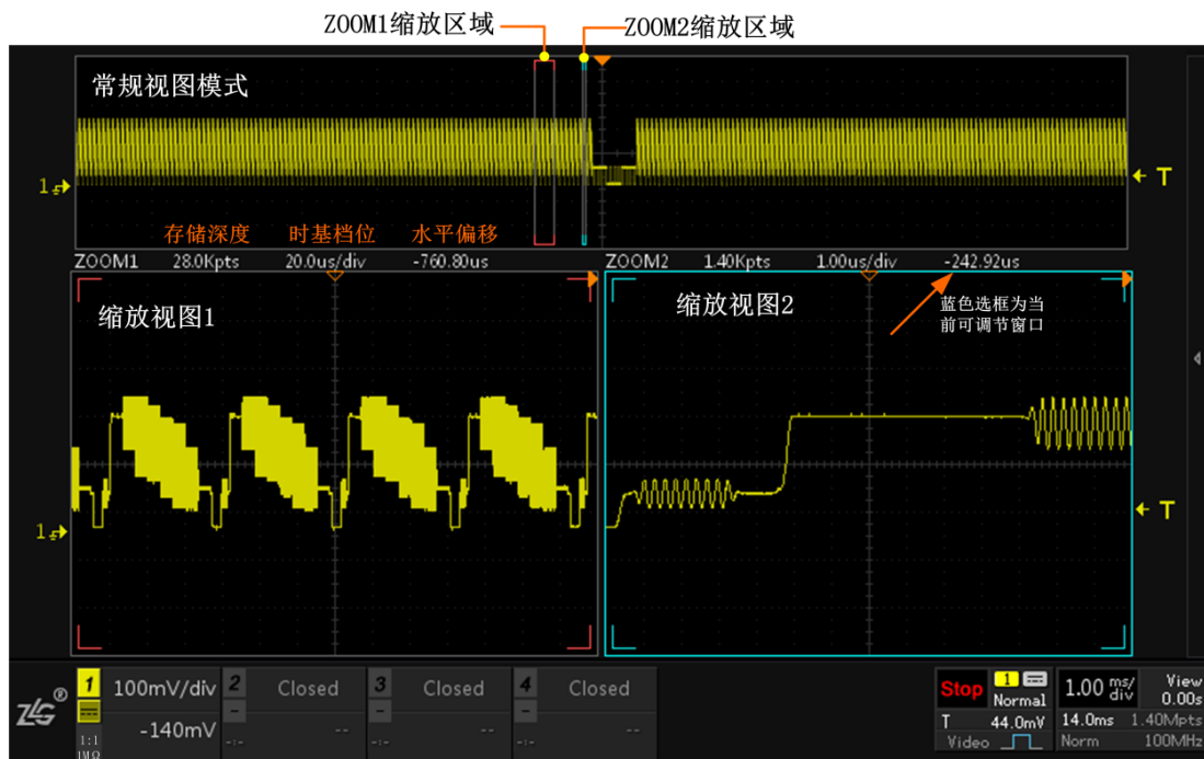
图 6.6 双 ZOOM 显示模式
