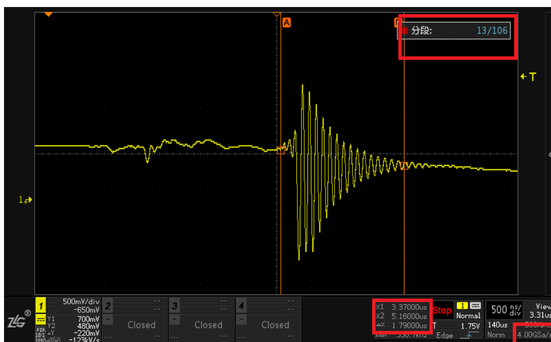
图 20.7 分段存储
