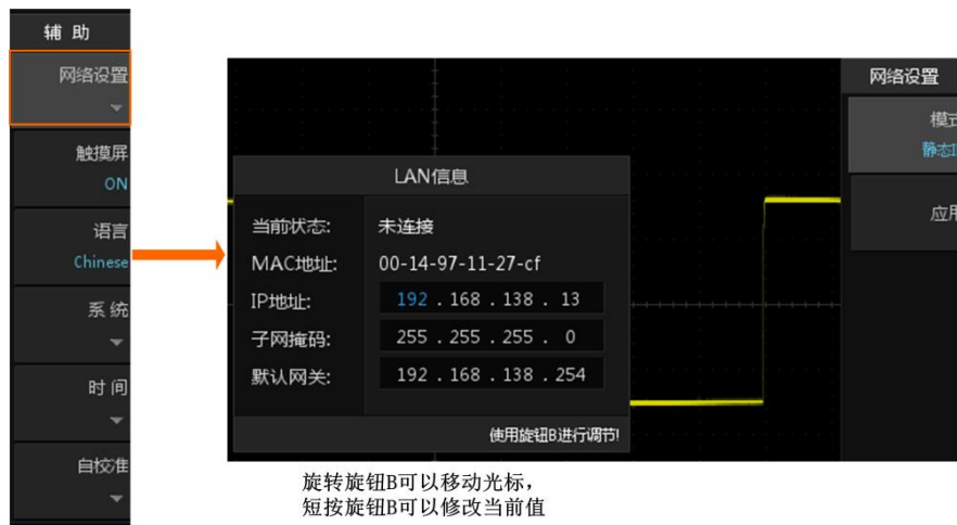
图 23.2 LAN 设置
