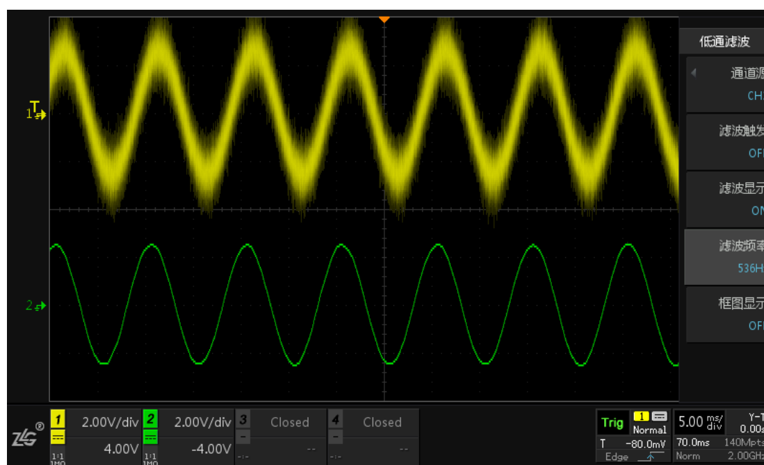
图 17.6 噪声滤波效果图
