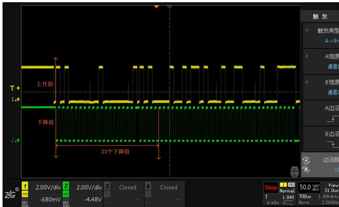
图 10.53 A->B 触发效果图
