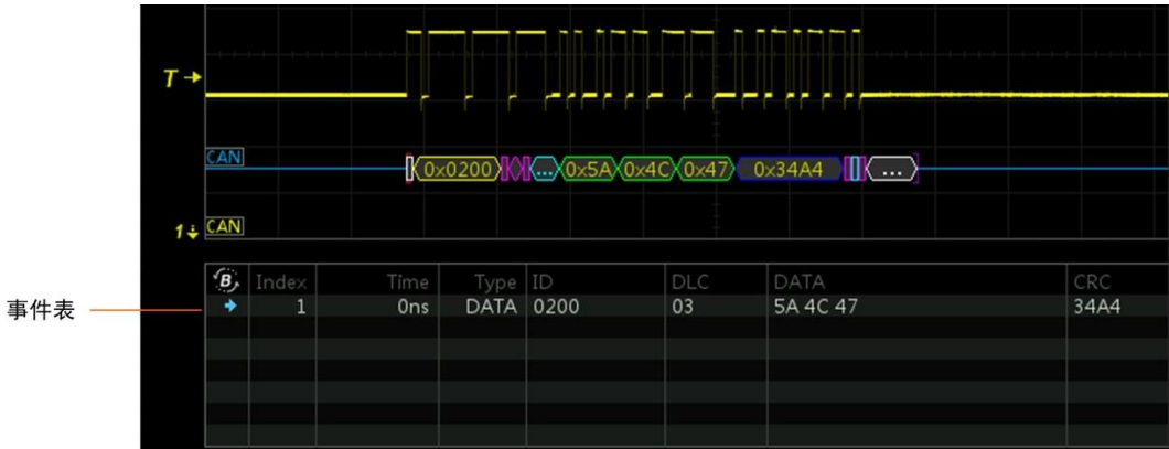
图 15.17 事件表
