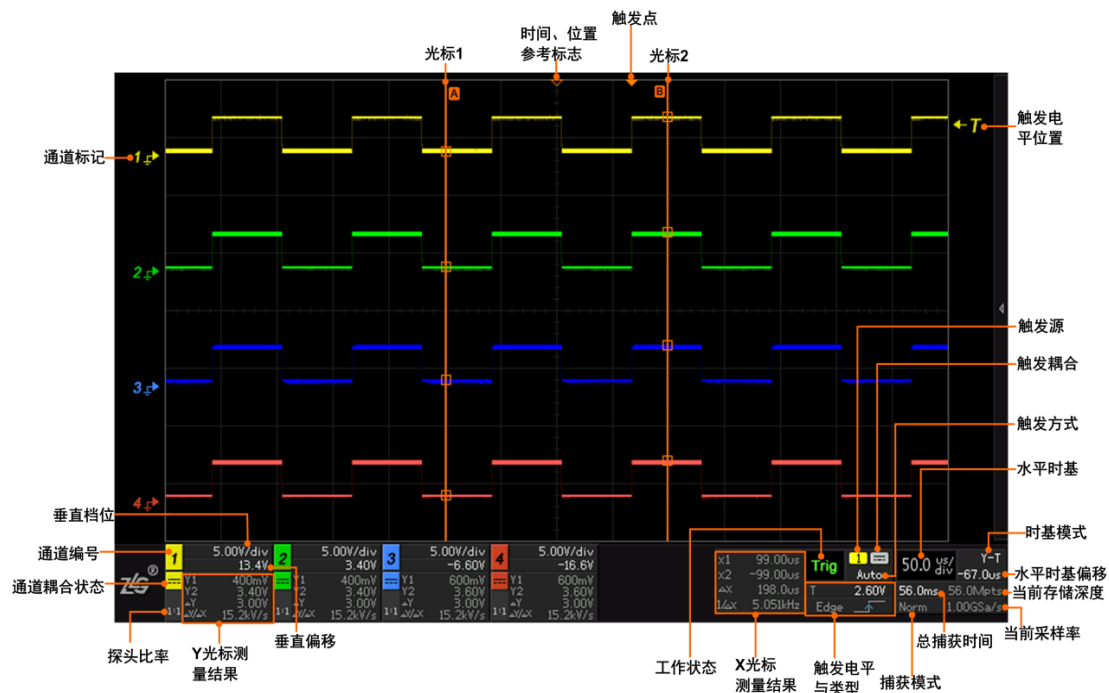
图 5.19 面板组件
