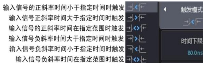
图 10.25 触发模式设置
