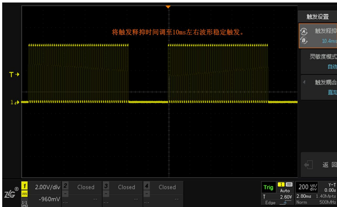
图 10.19 波形稳定显示
