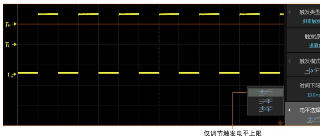
图 10.28 仅调节触发电平
