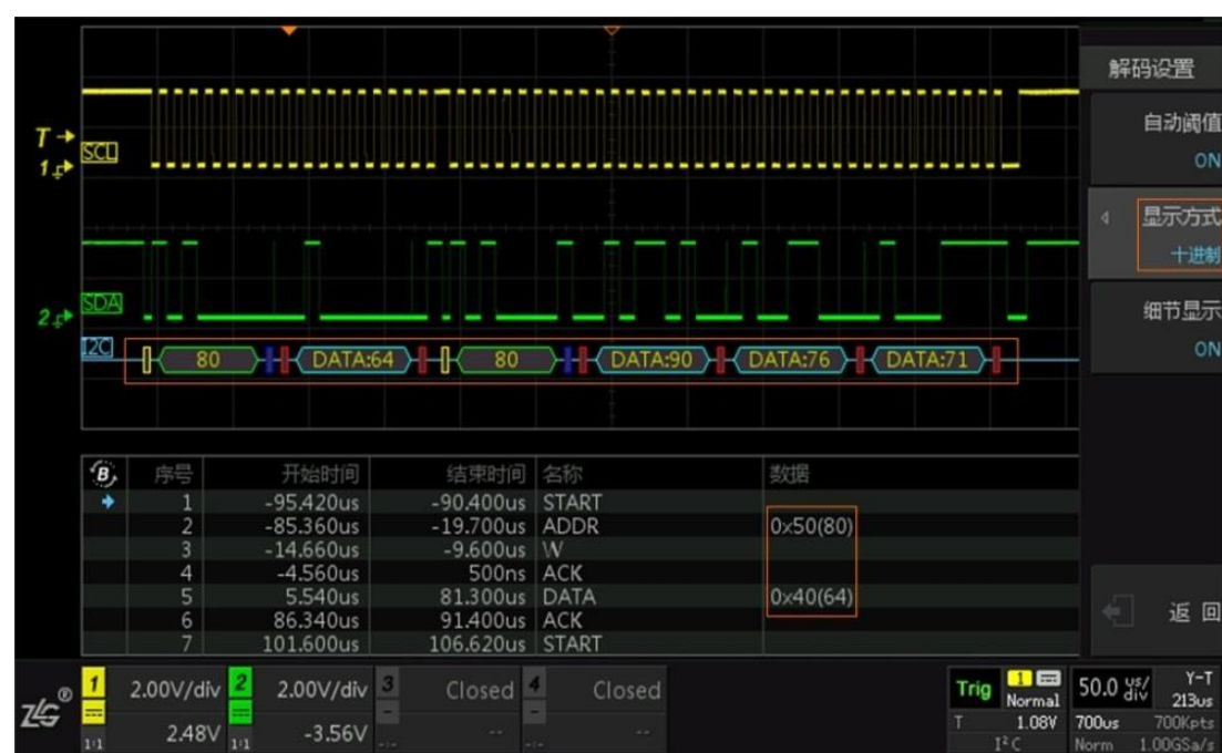
图 15.28 十进制显示
