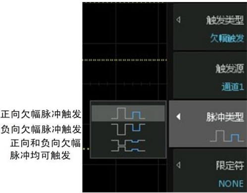
图 10.31 欠幅触发的脉冲类型
