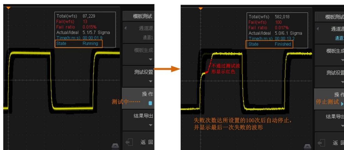
图 24.12 操作与停止
