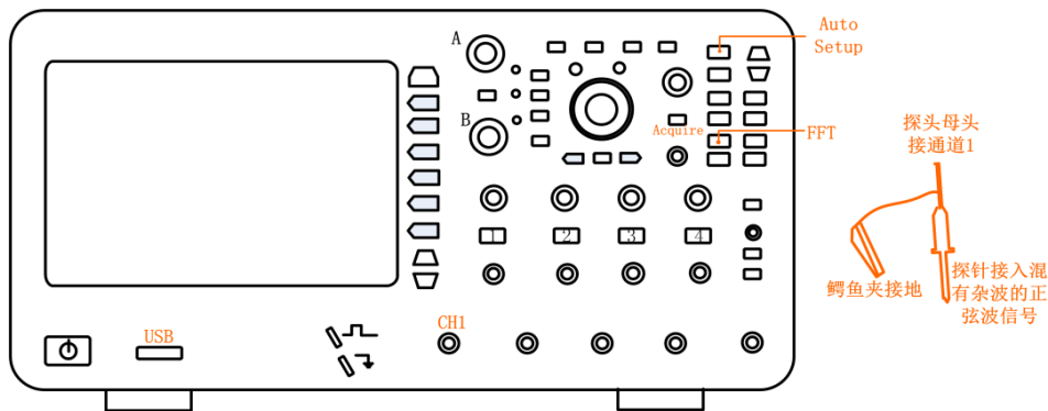
图 19.7 接入信号
