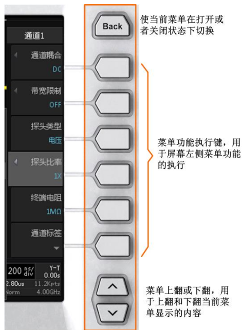
图 5.10 软键区
