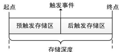
图 6.1 存储深度和可观察区间
