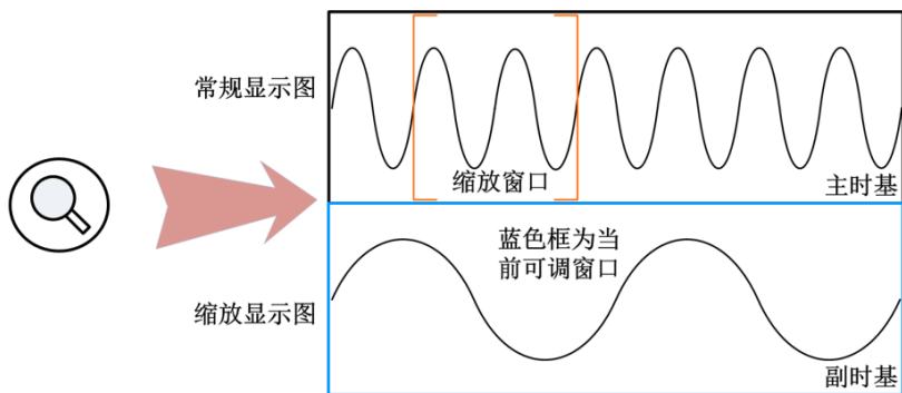
图 6.4 波形缩放
