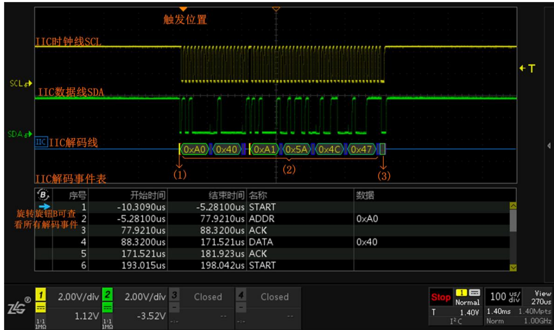
图 15.1 解码功能示意（ZDS4054 Plus 型）
